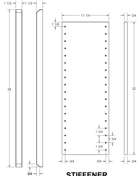
STIFFENER
