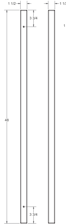
TOP SLAT
